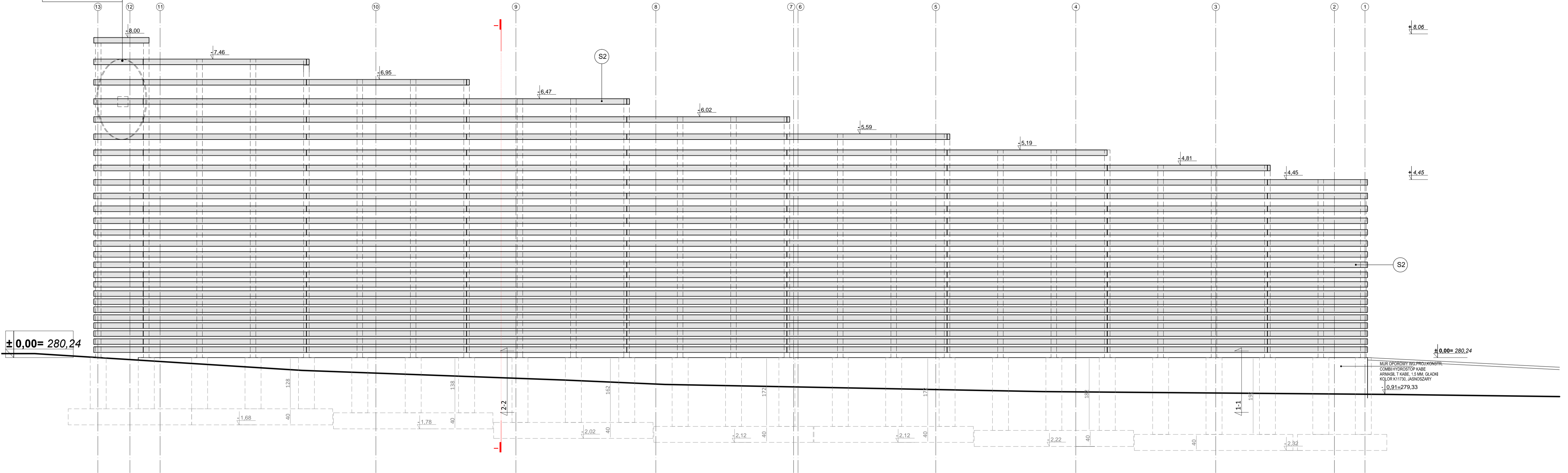
ELEWACJA ZACHODNIA
